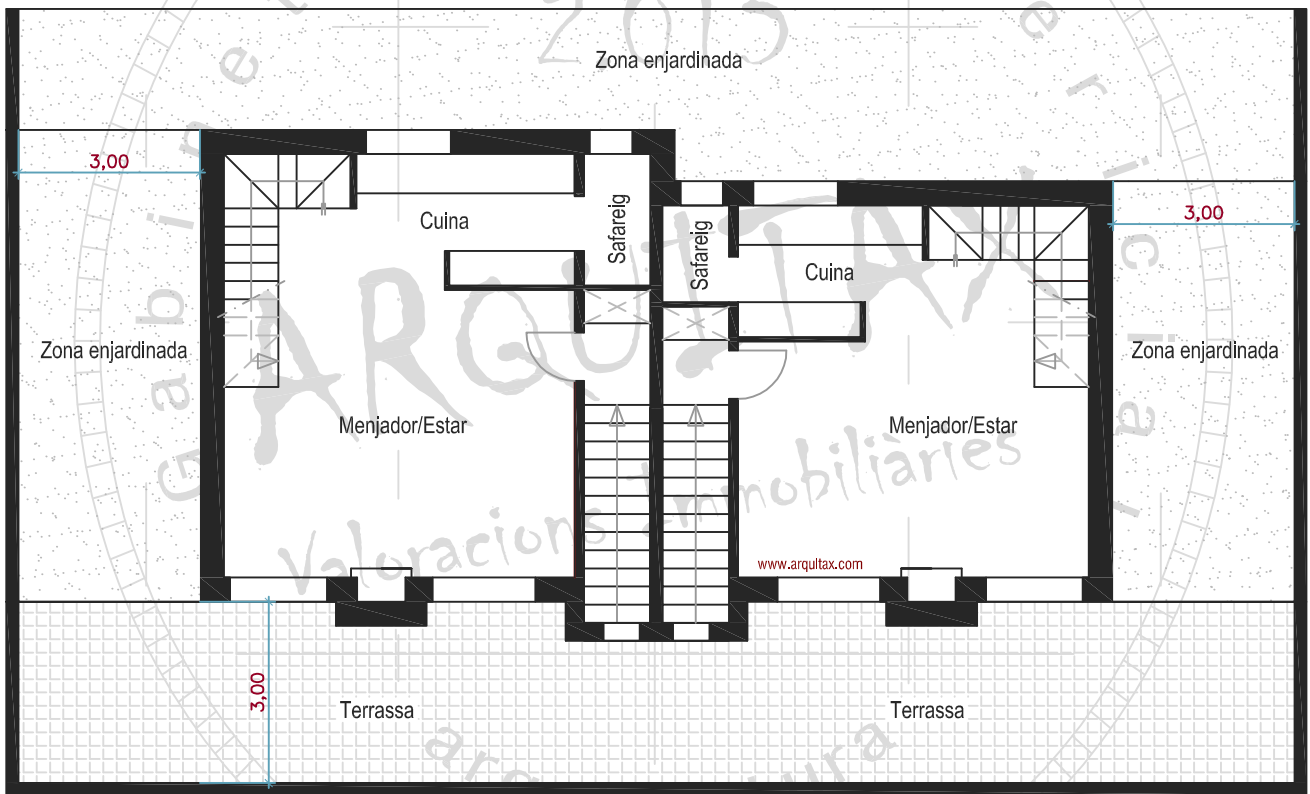
Planta Baixa
